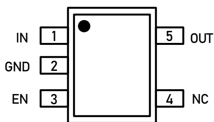
SOT23-5
