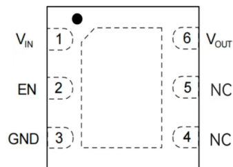
DFN 2x2 - 6L
